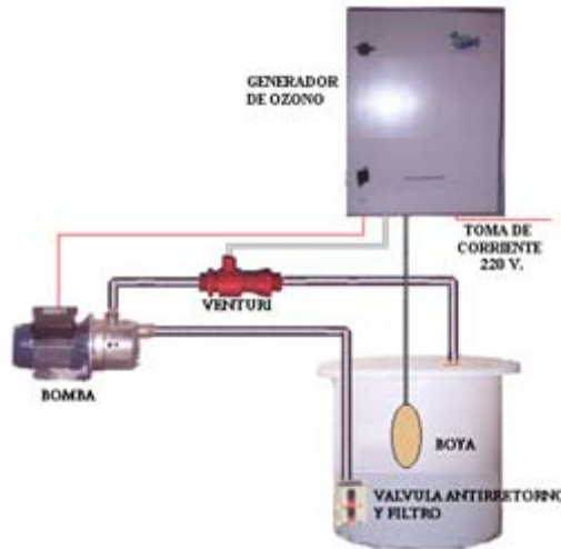
Detalle instalación en tanque de contacto con sonda de nivel
